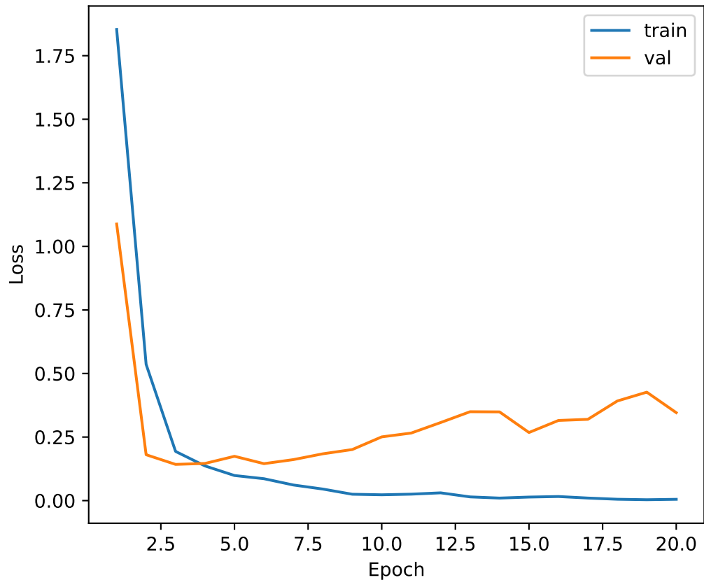
Loss per Epoch
